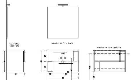
DISEGNO TECNICO
